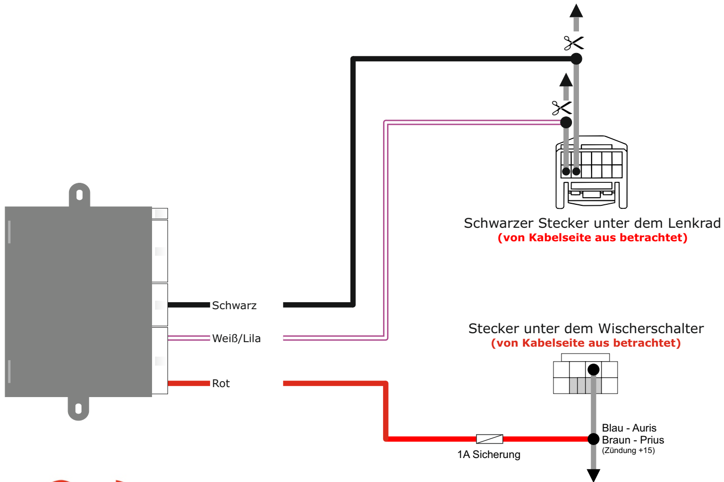
Die beiden Kabel in Position 1 & 2 schneiden. Schwarz und Weiß/Lila Kabel, wie gezeigt auflöten.
