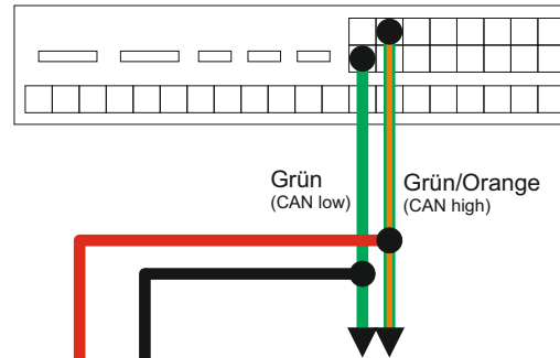
Stecker an ECU an der linken A-Säule (Von Kabelseite aus betrachtet)
