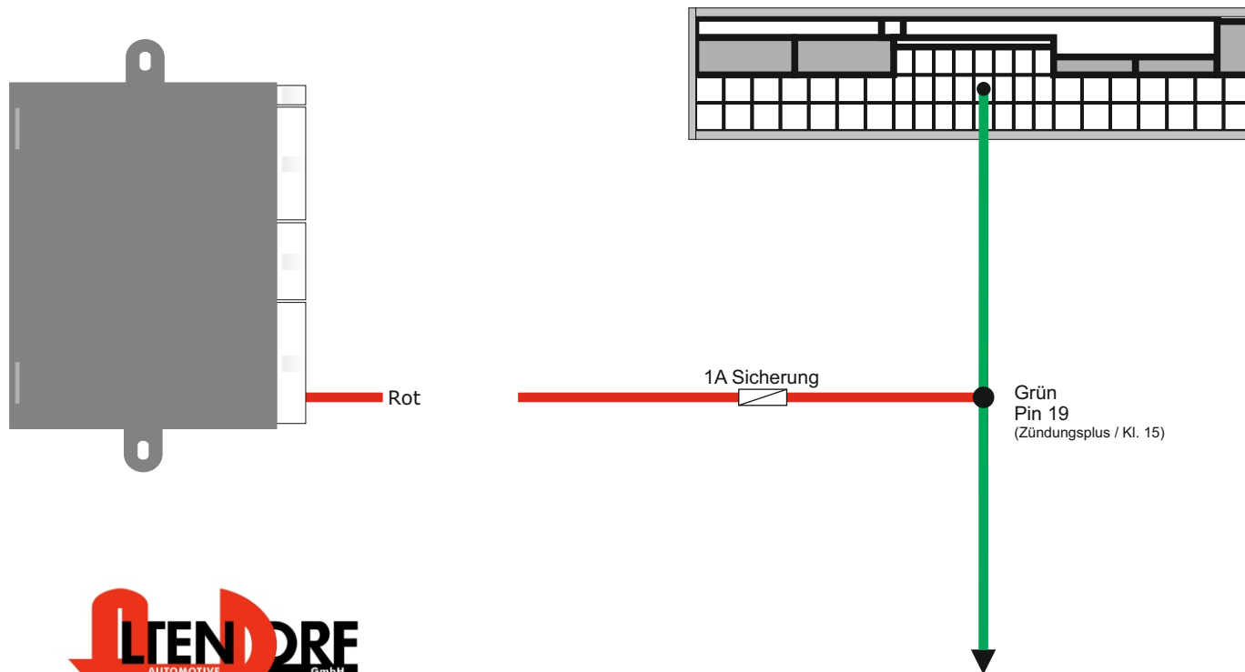
Stecker am Bordnetzsteuergerät (Abbildung von der Kabelseite)
