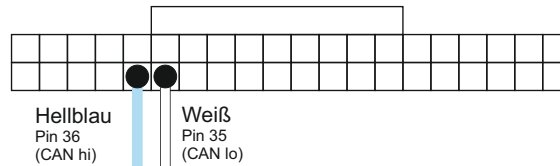
Weißer Stecker hinter dem Kombiinstrument (Aus Kabelsicht)
