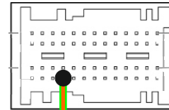
Blauer Stecker Sicherungskasten (Von der Kabelseite aus betrachtet)
