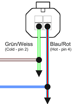
Stecker an Bremspedal (Von der Kabelseite ausbetrachtet)
