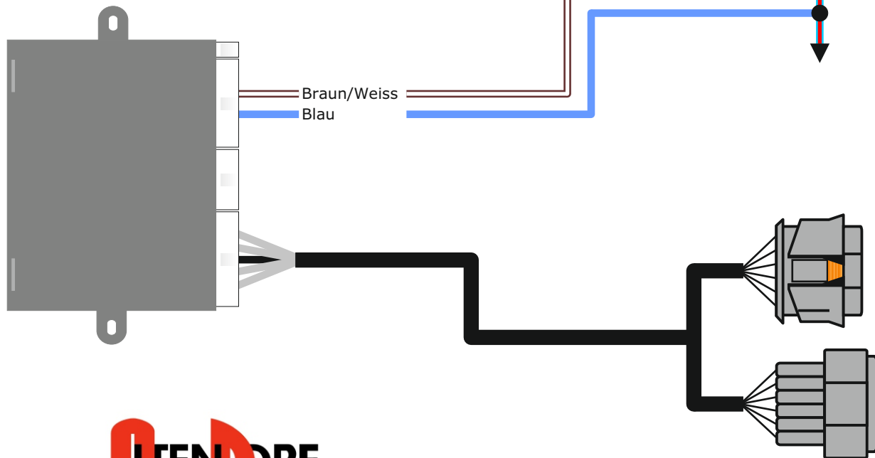
Stecker an Gaspedal
