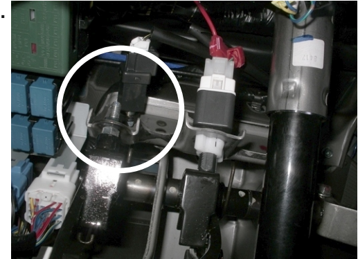
Anschlagbolzen entfernen und mitgelieferten Kupplungsschalter montieren und justieren.
