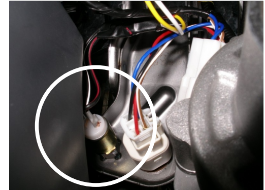
Diese Kabel nur bei Fahrzeugen mit man. Getriebe anschließen.
