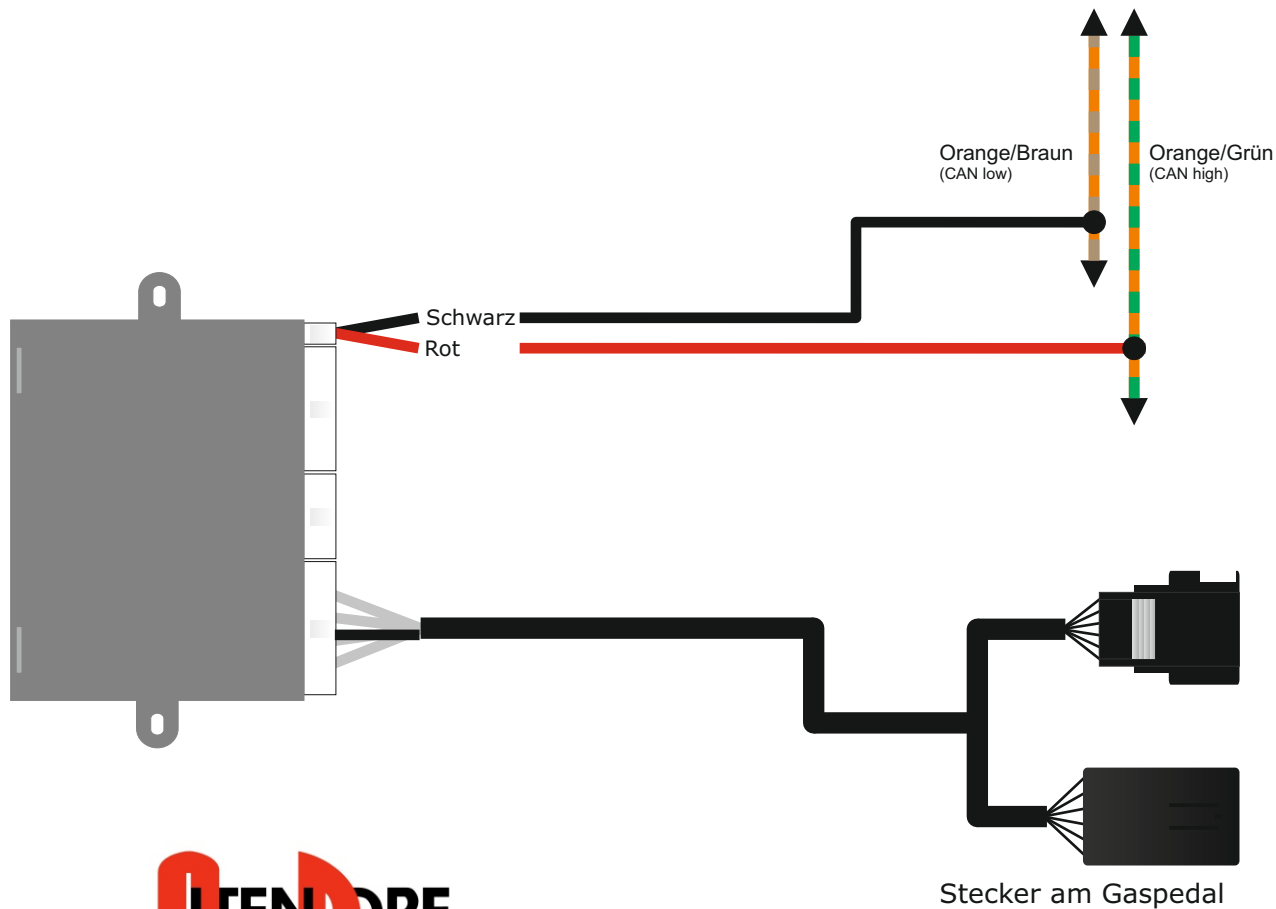
Hellbrauner Stecker am BCM T 52 C (verdrillte Leitungen i.d.R. Pin 15 & 16)
