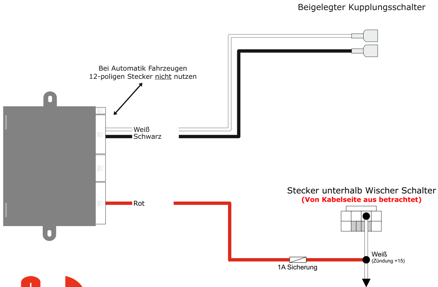
Den beigelegten Kupplungsschalter so justieren das der Pedal Stop analog der originalen Position des Anschlags ist
