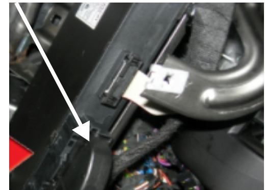
Autozugangssystem befindet sich hinter/ unter dem Lichtschalter. 41-pin Stecker.
