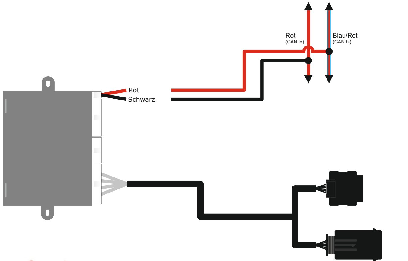
Kabelbaum an der A-Säule Fahrerseite
