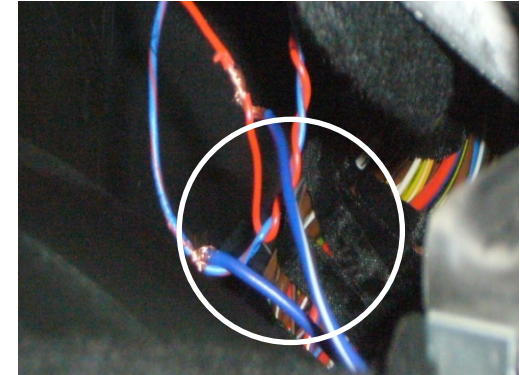
CAN Kabel sind alternativ hinter dem Handschuhfach
