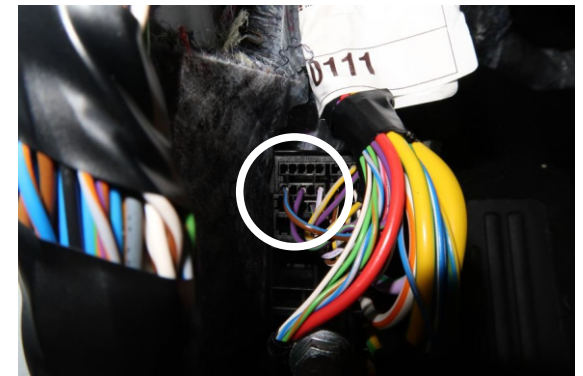
Kabel im Stecker am Kabelbaum an der linken A-Säule
