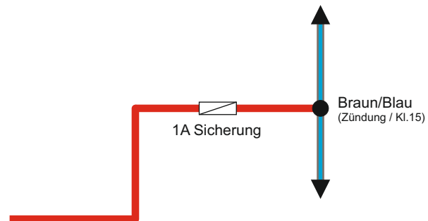
Kabel im Stecker am Kabelbaum an der linken A-Säule
