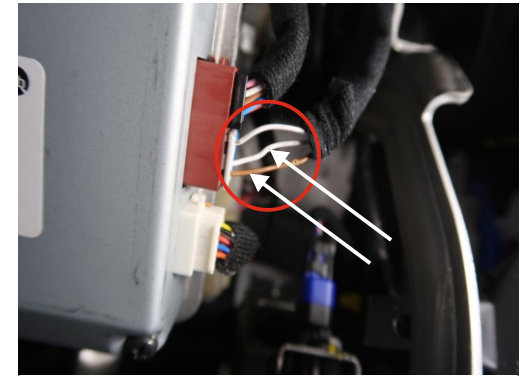
Stecker an ECU für Servolenkung.
