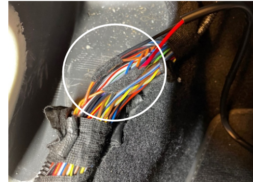
CAN bus Kabel befinden sich im Kabelbaum von der A-Säule und rückwärts
