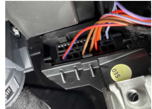
OBD Stecker +15 (Zündung)
