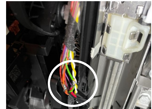
CAN Kabel unterhalb der Lenksäule. Grünes Kabel kann auch Orange/Grün sein.
