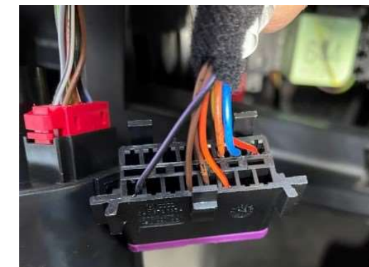
Pin 1 OBD Stecker
