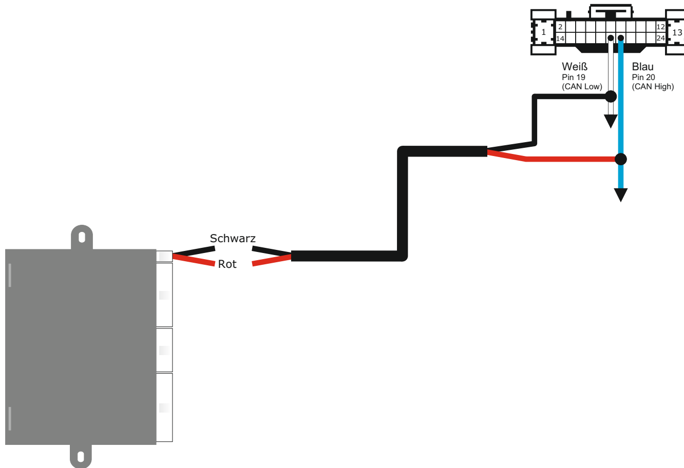
Gateway-Stecker hinter dem OBD-Stecker
