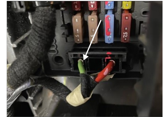
Der Stecker befindet sich im unteren Teil des Sicherungshalters (unter dem Handschufach).
