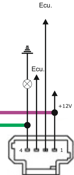
Bremslichtschalter. (Aus Kabelsicht)
