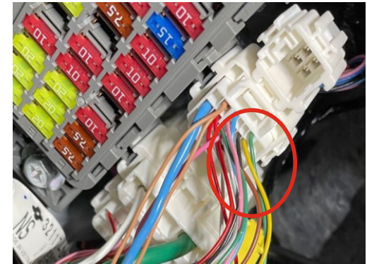
CAN Bus Kabel befinden sich links neben dem Bremspedal, in der Nähe des Sicherungskastens.
