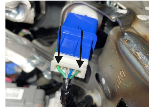
Grün und Lila Kabel auf die zwei grünen Kabel des Bremslichtschalters löten. Lila Pin 1, Grün Pin 4.
