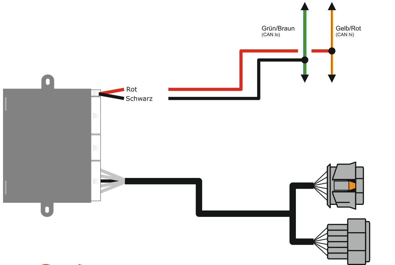
Stecker hinter der Plastikabdeckung der A-Säule. (Kabel sind verdreht)
