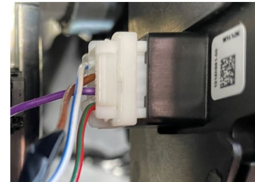
Stecker am OE Bedienelement.
