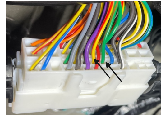
Stecker hinter der Plastikabdeckung der A-Säule. (Kabel sind verdreht)
