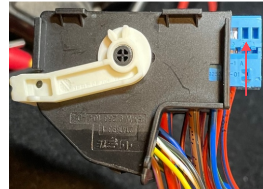
BCM in der rechten A-Säule Trennen Sie den Stecker, lösen Sie den blauen Teil und pinnen Sie den Pin in Pin 2. ( Zündung)
