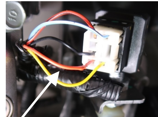
Bremslichtschalter
