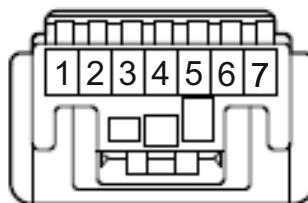
Stecker am Bremslichtschalter (Aus Kabelsicht)
